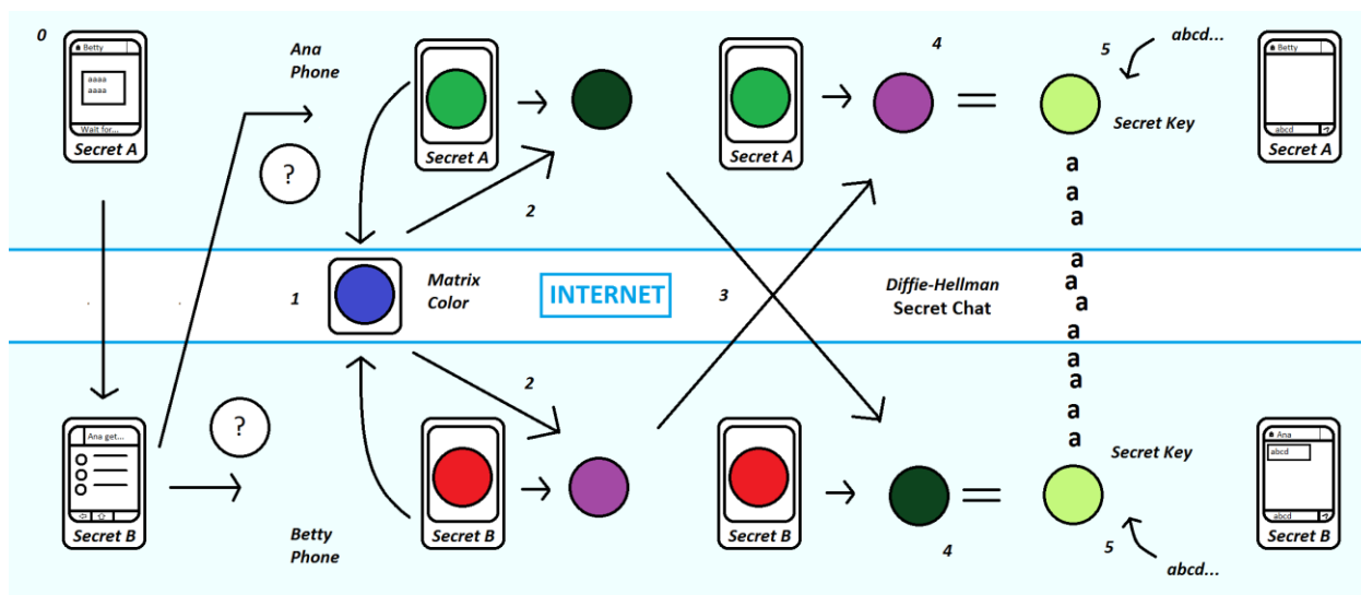
Рисунок 1 – Упрощенная схема шифрования MTProto
