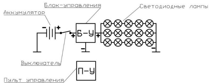
Рисунок 1 – Схема подключения
