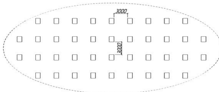
Рисунок 2 – Схема расположения свай
